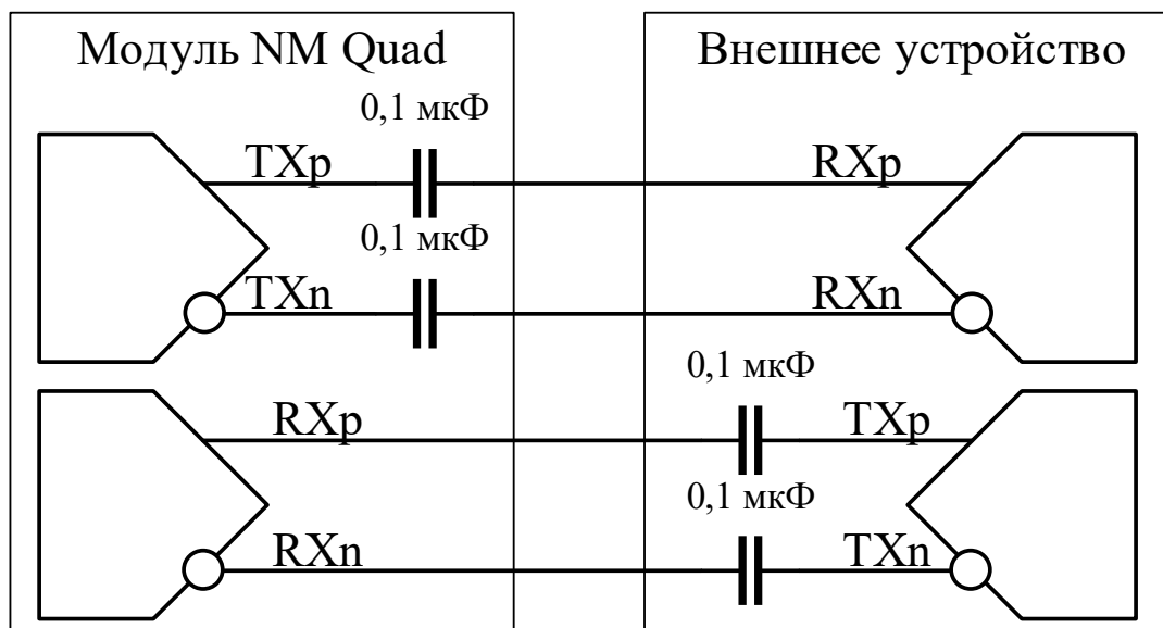
Рисунок 2.6 – Согласование передающей и приёмной линий
