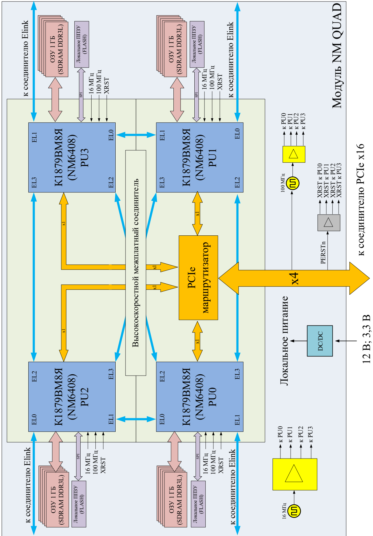
Рисунок 1.4 – Функциональная схема Модуля NM Quad
