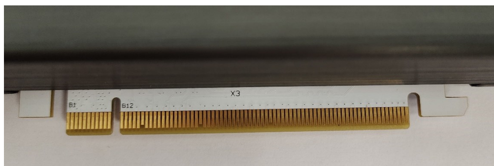
Рисунок 2.2 – Соединитель X3 (ряд В) интерфейса PCIe x4 модуля NM Quad
