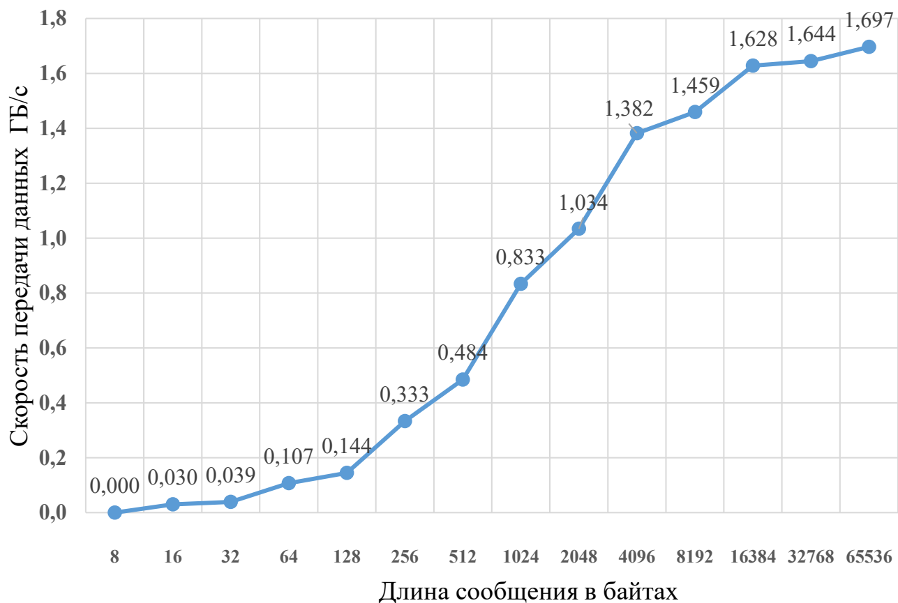
Рисунок 2.7 – Зависимость скорости передачи данных от длины сообщения
