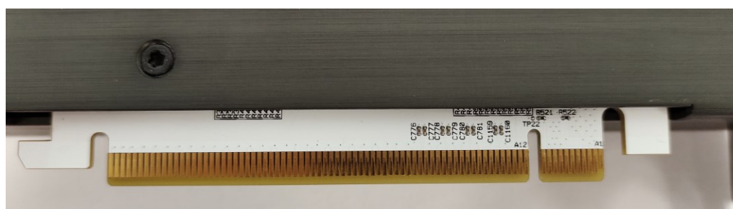
Рисунок 2.3 – Соединитель X3 (ряд А) интерфейса PCIe x4 модуля NM Quad
