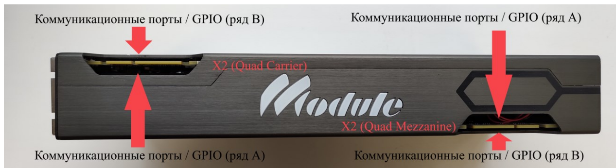
Рисунок 2.1 – Соединители X2 модуля NM Quad
